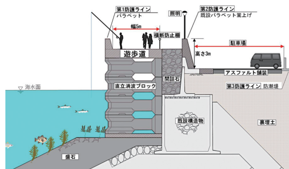
▲ 護岸復旧断面イメージ図
